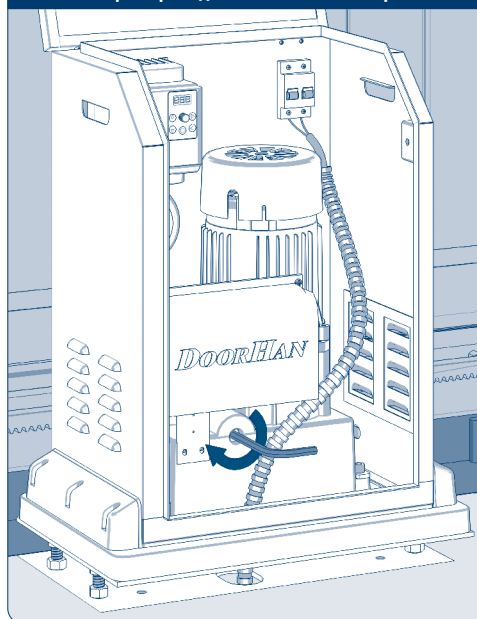
Рис. 4. Возврат привода в автоматический режим
