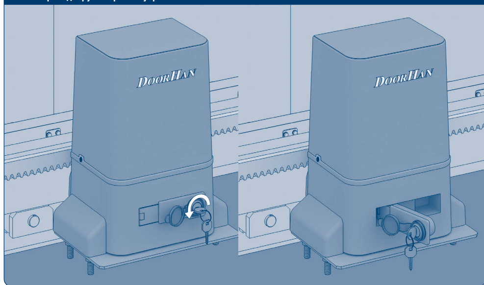
Рис. 1. Перевод в ручной режим управления
