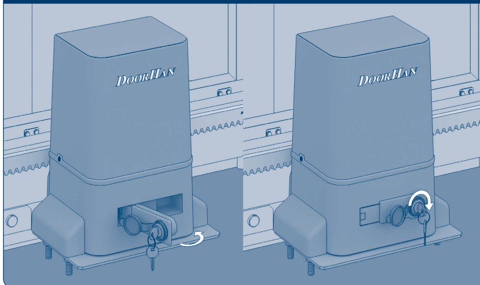
Рис. 2. Возврат привода в автоматический режим
