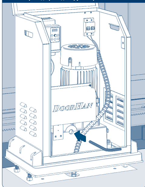
Рис. 3. Перевод привода в ручной режим
