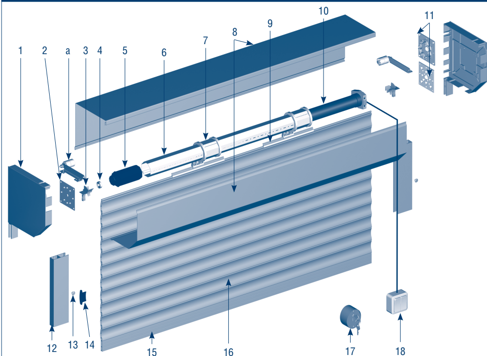
Рис. 3.1.4. Роллетные системы с электроприводом
