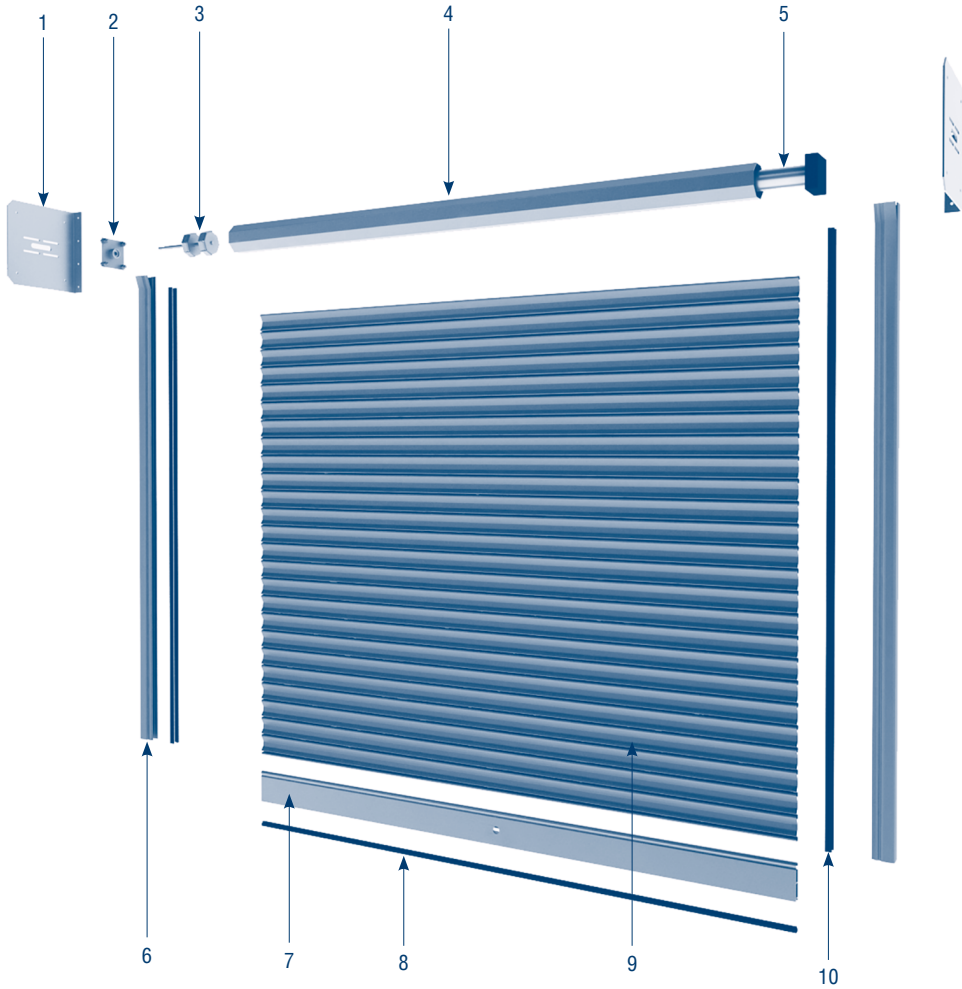
Рис. 3.2.2. Рулонные ворота с внутривальным приводом
