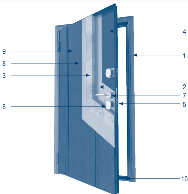
Рис. 1. Конструкция дверей
